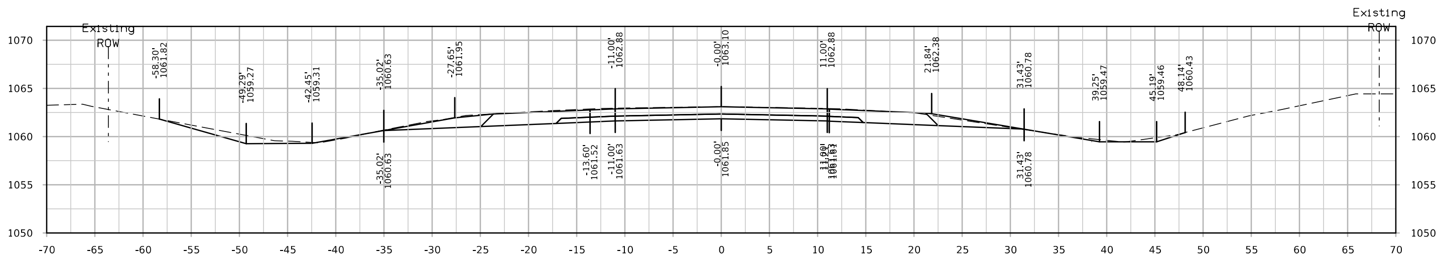
STA. 7182+50.00
